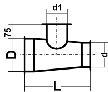
L = d1 + 190 Abzweiger 90° direkt reduziert réduit direct
