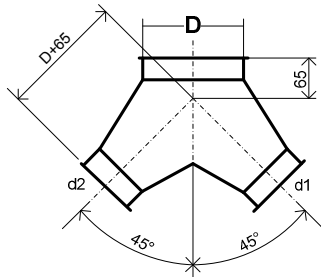
Hosenrohr 45° Culotte 45°
