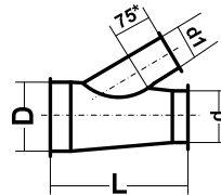
L = (d1:0,5) + 270 Abzweiger 30° direkt reduziert / réduit direct *150mm bei Flanschbord / avec bord pour flasque
