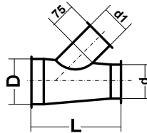
L = (d1:0,7) + 190 Abzweiger 45° direkt reduziert réduit direct
